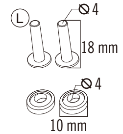
2 pcs UDG rivet and washer
